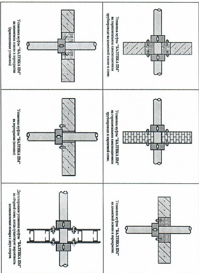
Схема установки 1
